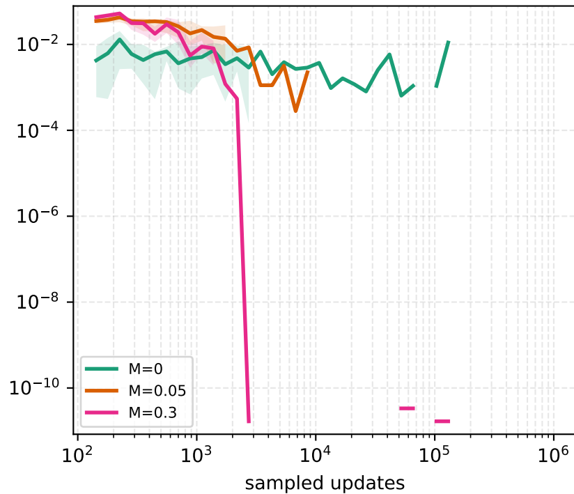
SIS
