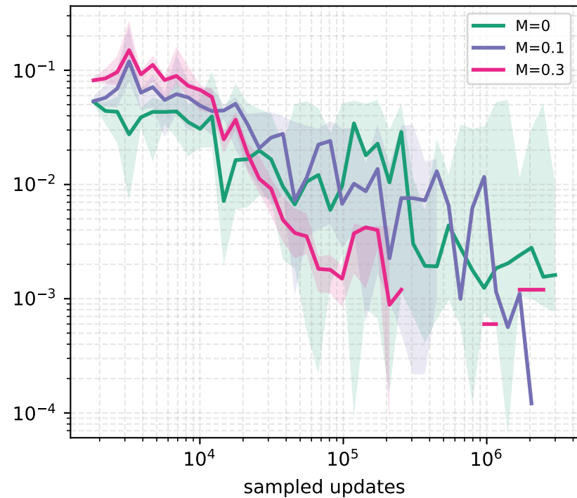
SEIR
