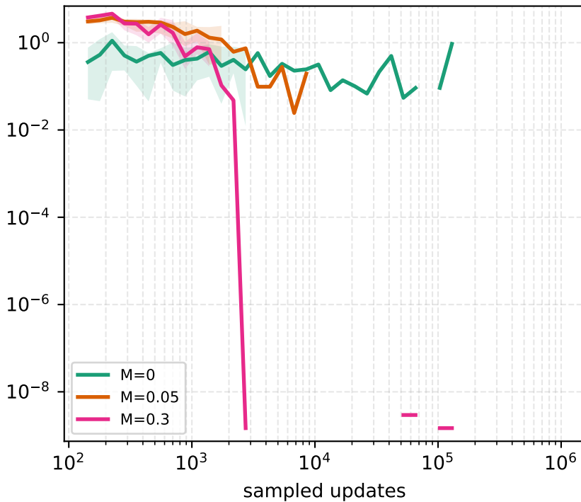
SIS
