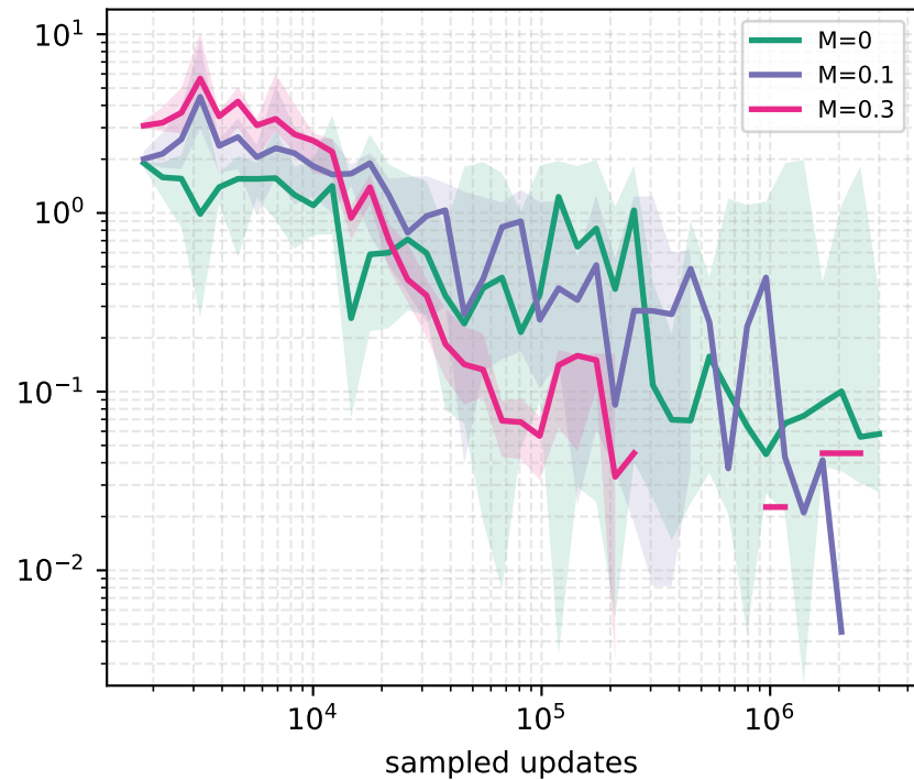
SEIR
