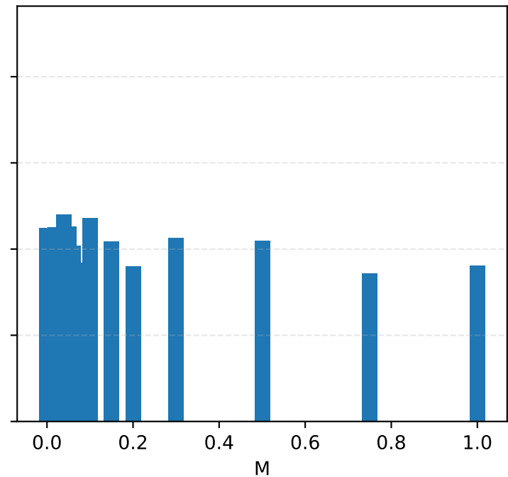
SEIR
