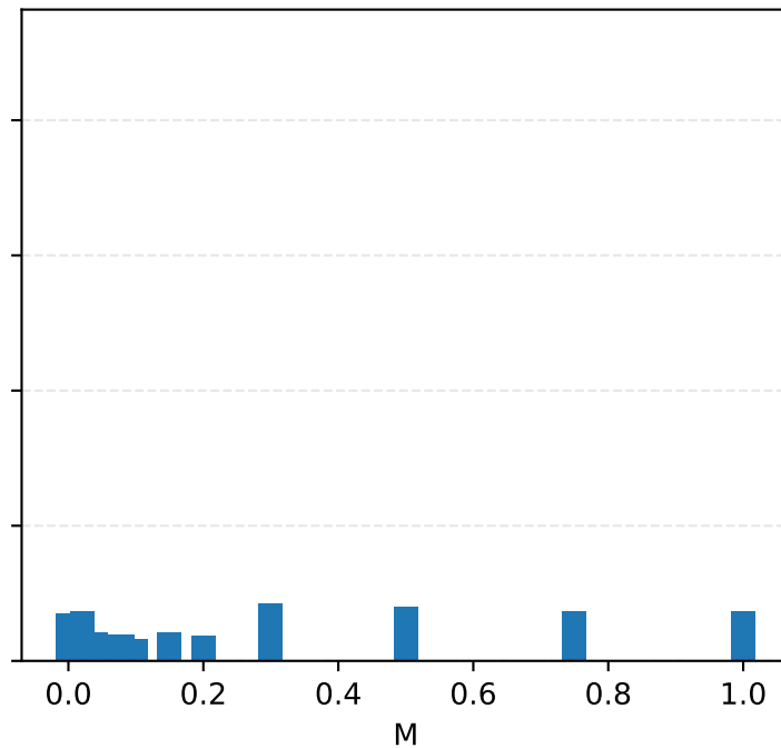
SIS
