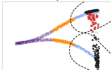
Curly-FM
