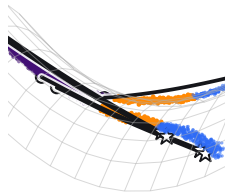
Curly-FM
