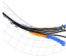
MFM / LAND
