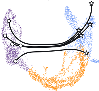
MFM / LAND
