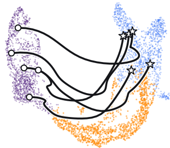
Curly-FM
