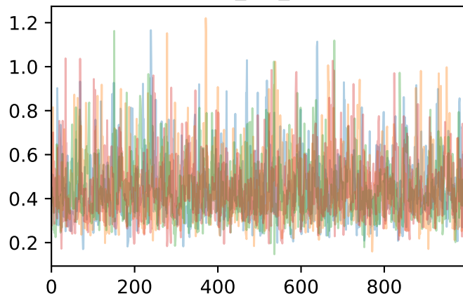
sigma_log_alpha
