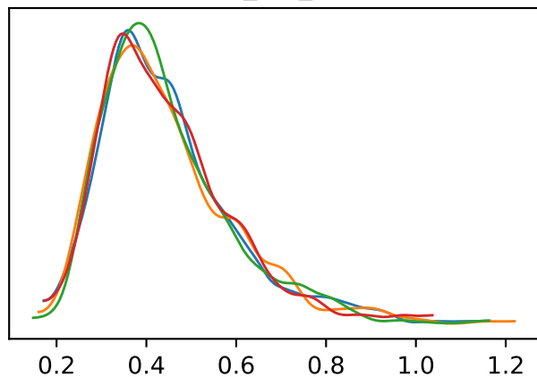
sigma_log_alpha
