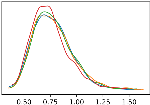
sigma_log_alpha
