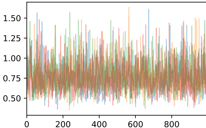
sigma_log_alpha
