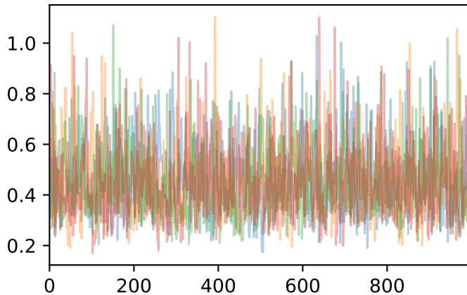
sigma_log_alpha
