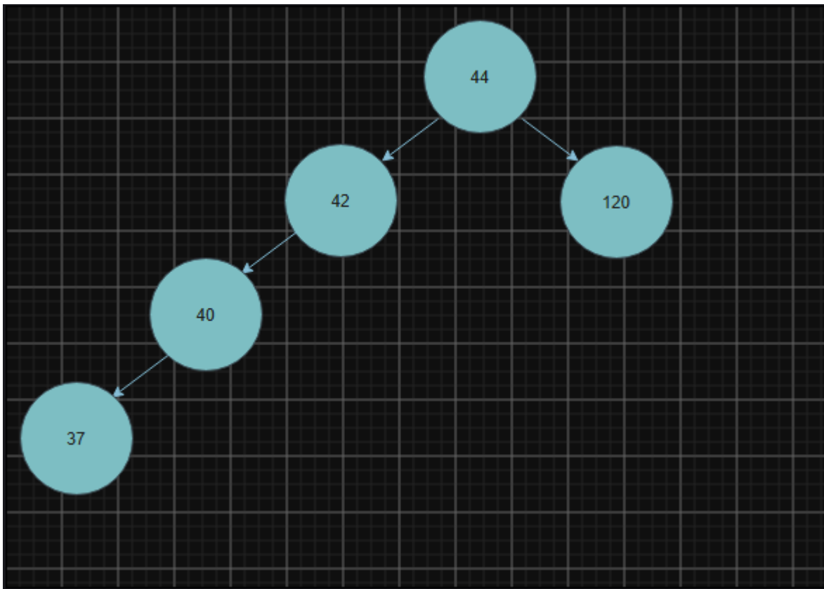
Rotación Simple Izquierda sobre 42.
