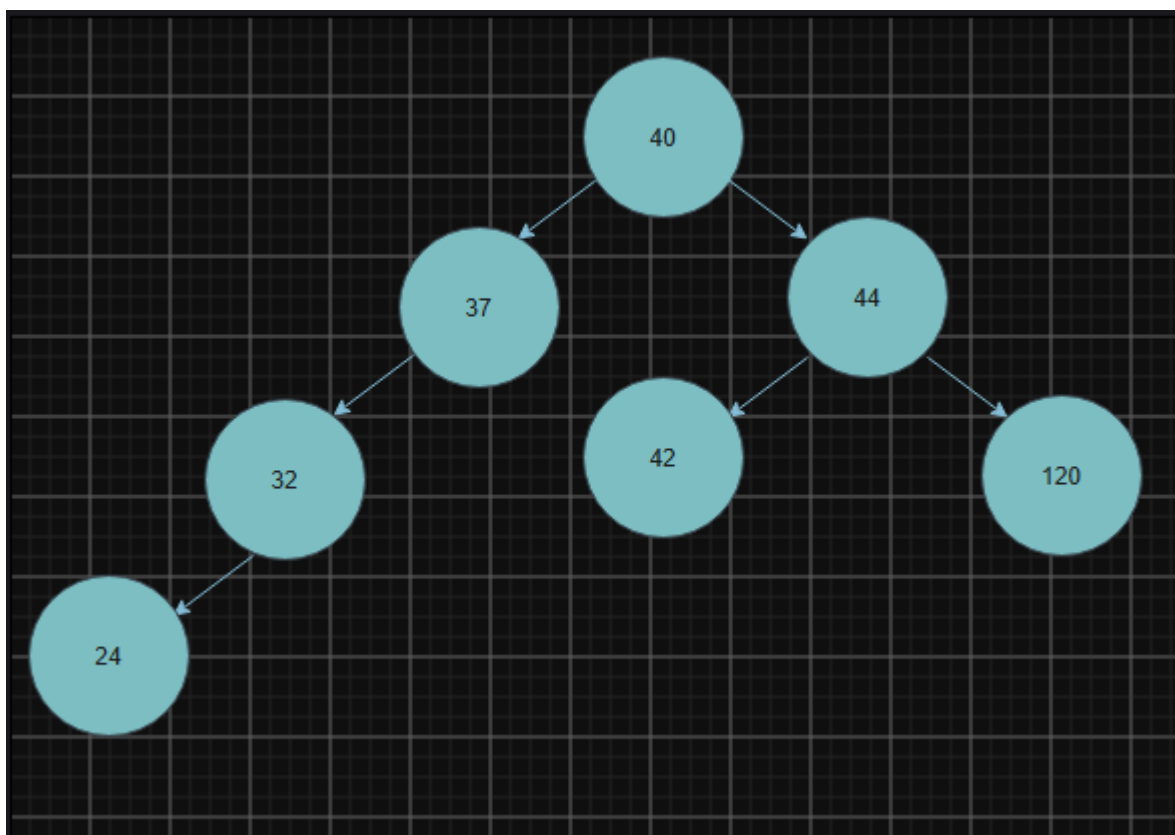
Rotación Simple Izquierda en 37
