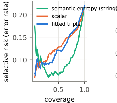
TriviaQA
