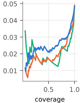
SciQ-MC
