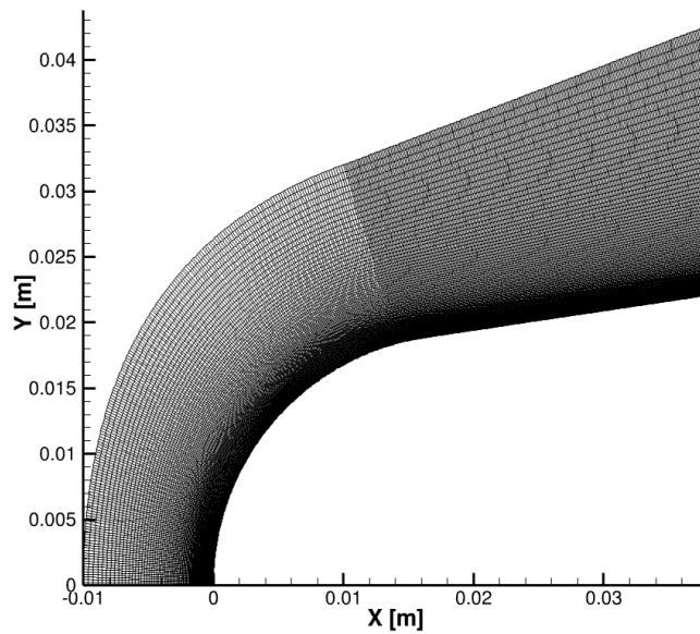
(b) IRV-2 mesh
