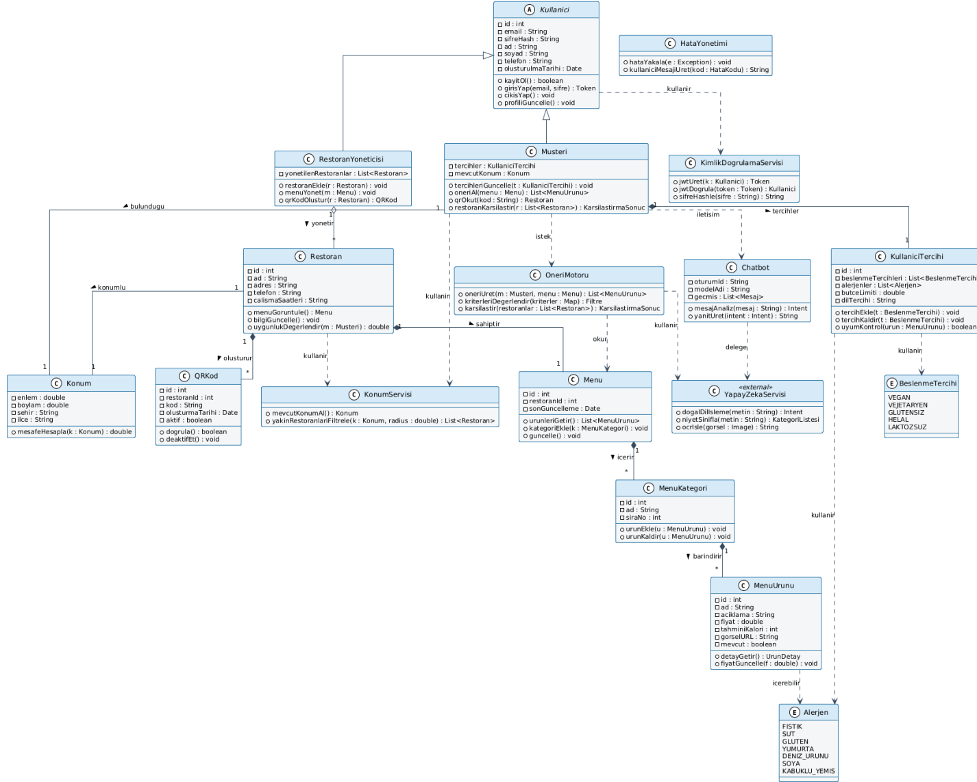
Pick A Bite — Sınıf Diyagramı
