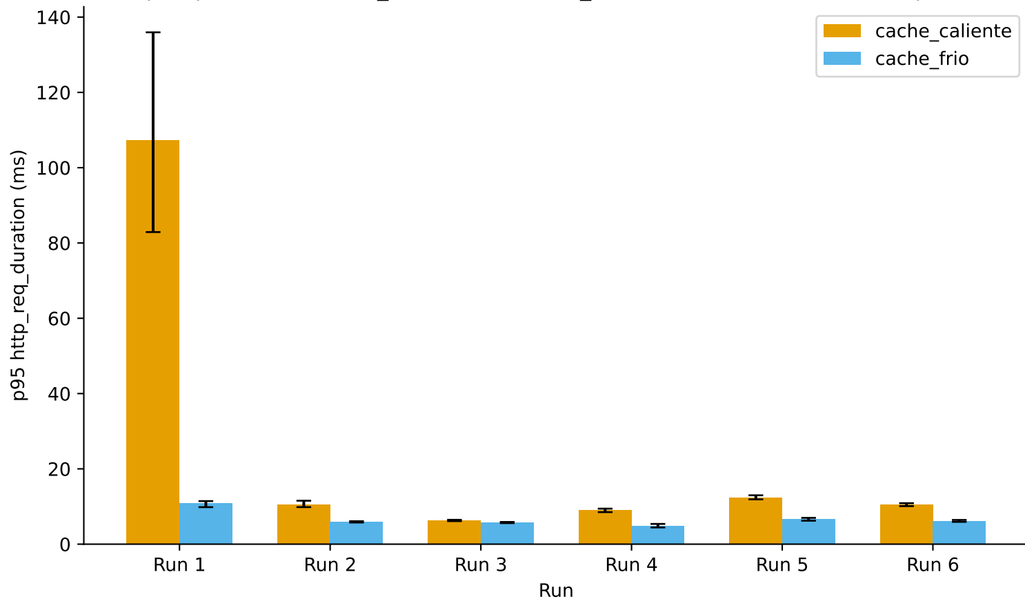
p95 per run — cache_caliente vs cache_frio (error bars: 95% bootstrap CI)
