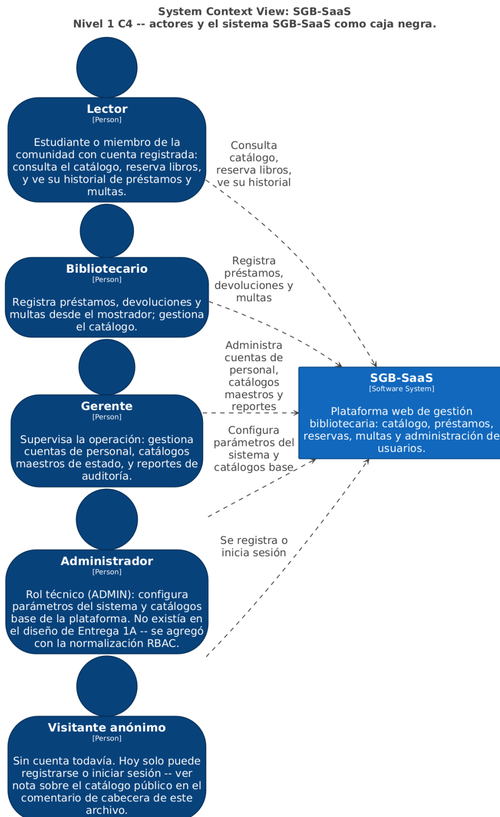
Figura 6.1: Modelo C4, Nivel 1 (Contexto): los cinco actores del sistema y sus interacciones con SGB-SaaS como caja negra. Exportado automáticamente desde workspace.dsl .
