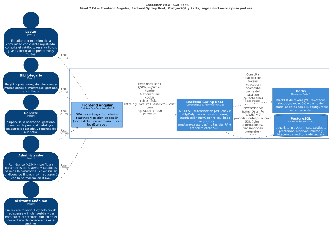
Figura 6.2: Modelo C4, Nivel 2 (Contenedores): Frontend Angular, Backend Spring Boot, PostgreSQL y Redis, alineados 1:1 con docker-compose.yml . Exportado automáticamente desde workspace.dsl .
