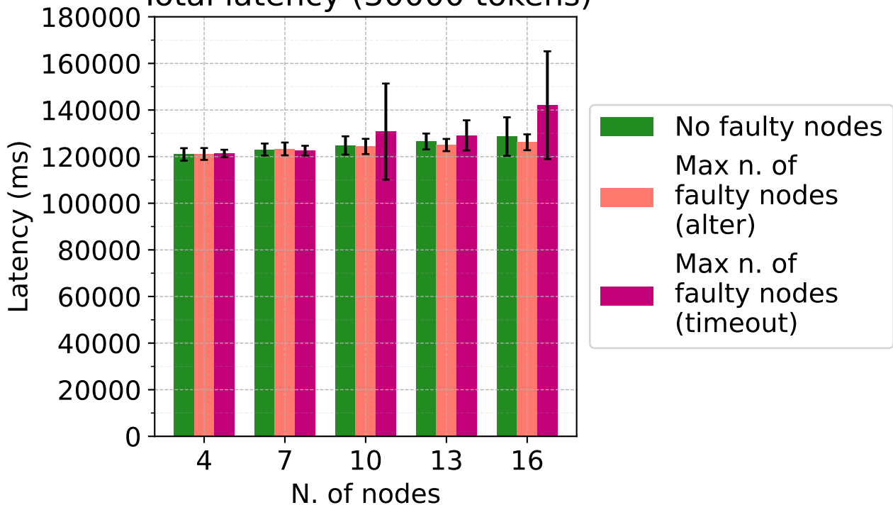
Total latency (30000 tokens)
