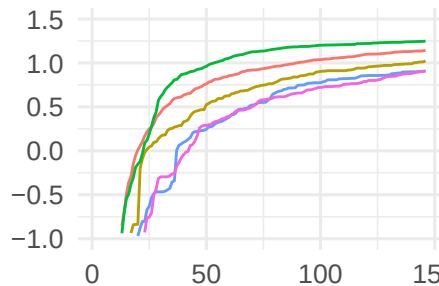
rbv2_xgboost 1501
