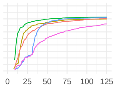
rbv2_xgboost 12
