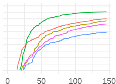
rbv2_xgboost 12
