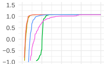
rbv2_xgboost 1501
