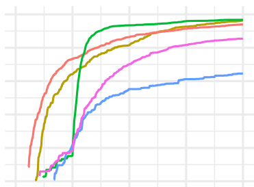
rbv2_xgboost 12
