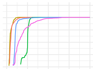
rbv2_xgboost 40499
