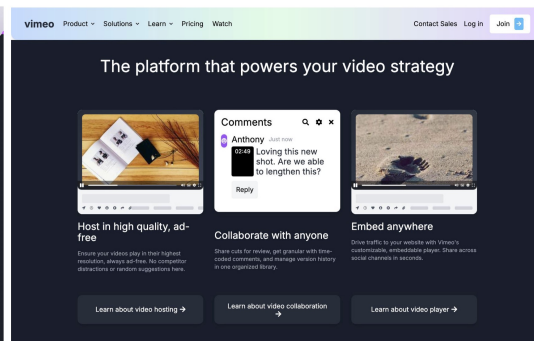
UI2Code N
