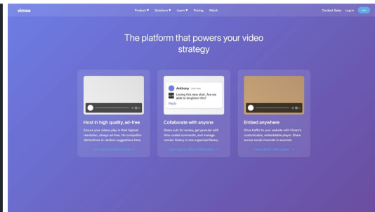
Claude-4-Sonnet
