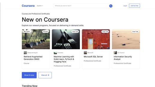
Claude-4-Sonnet
