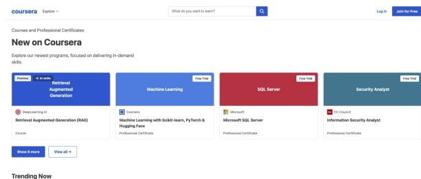
Gemini-2.5-Pro
