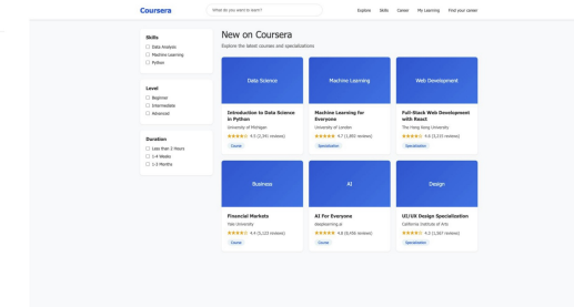
Claude-4-Sonnet
