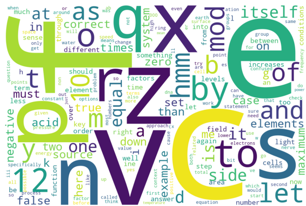
(a) Layer 75
