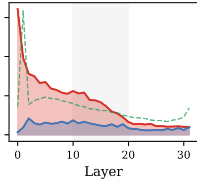
Mistral-7B V/O:Q/K = 3.66×
