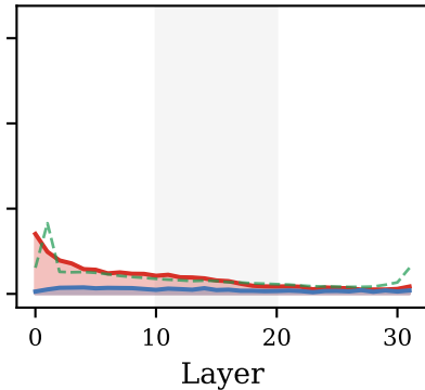
Llama-3.1-8B V/O:Q/K = 3.91×
