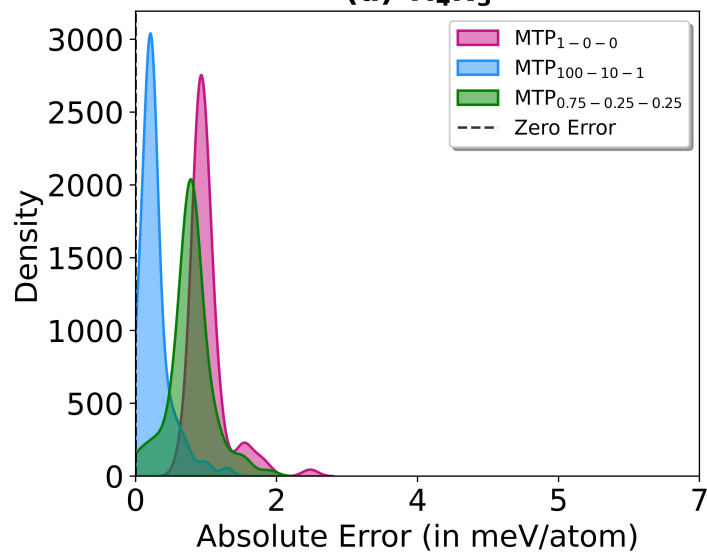
(d) Ti_4N_3
