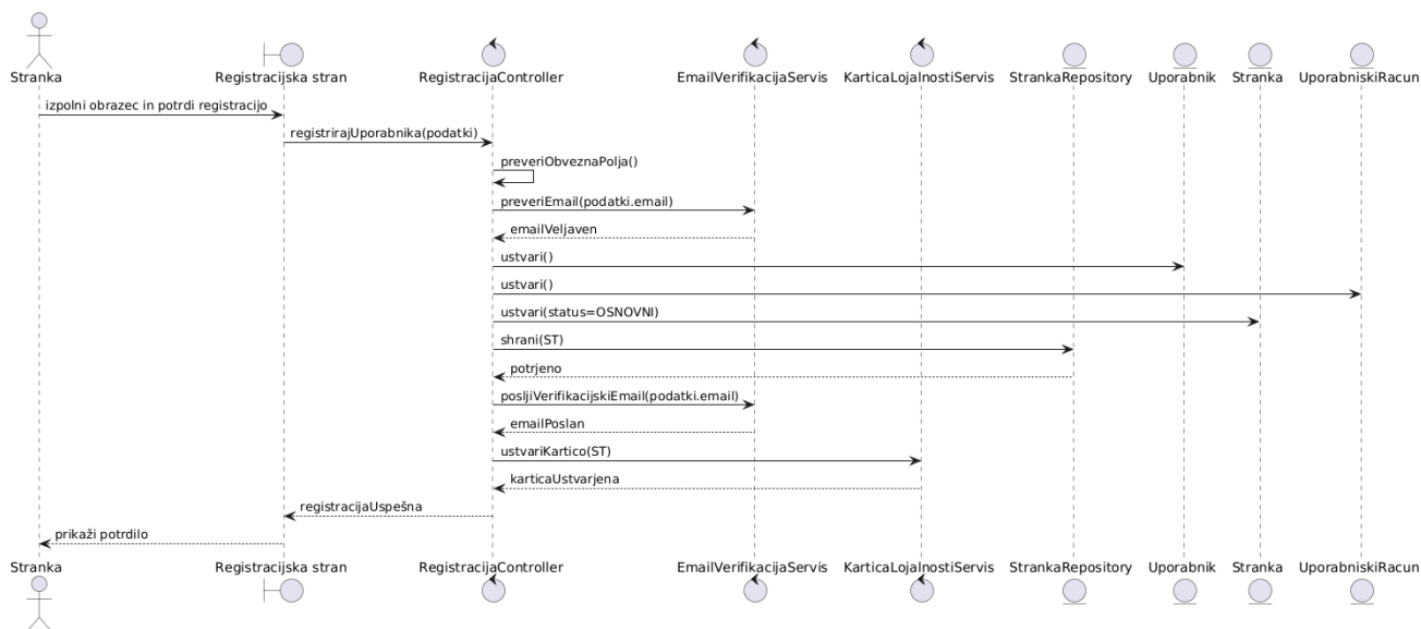
Diagram zaporedja - registracija uporabnika
