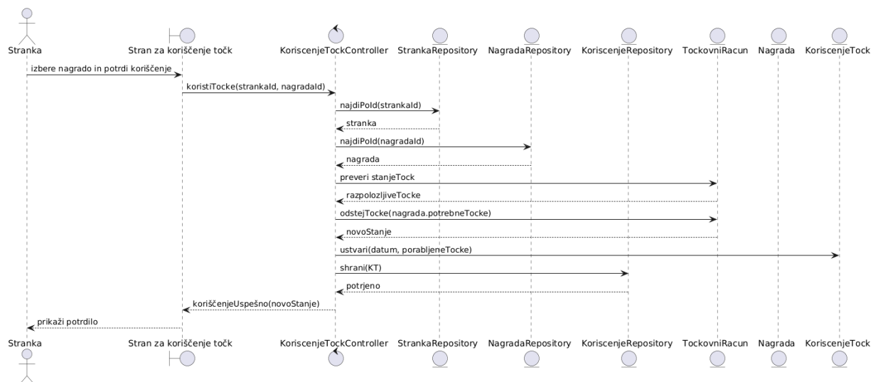
Diagram zaporedja - koriščenje točk
