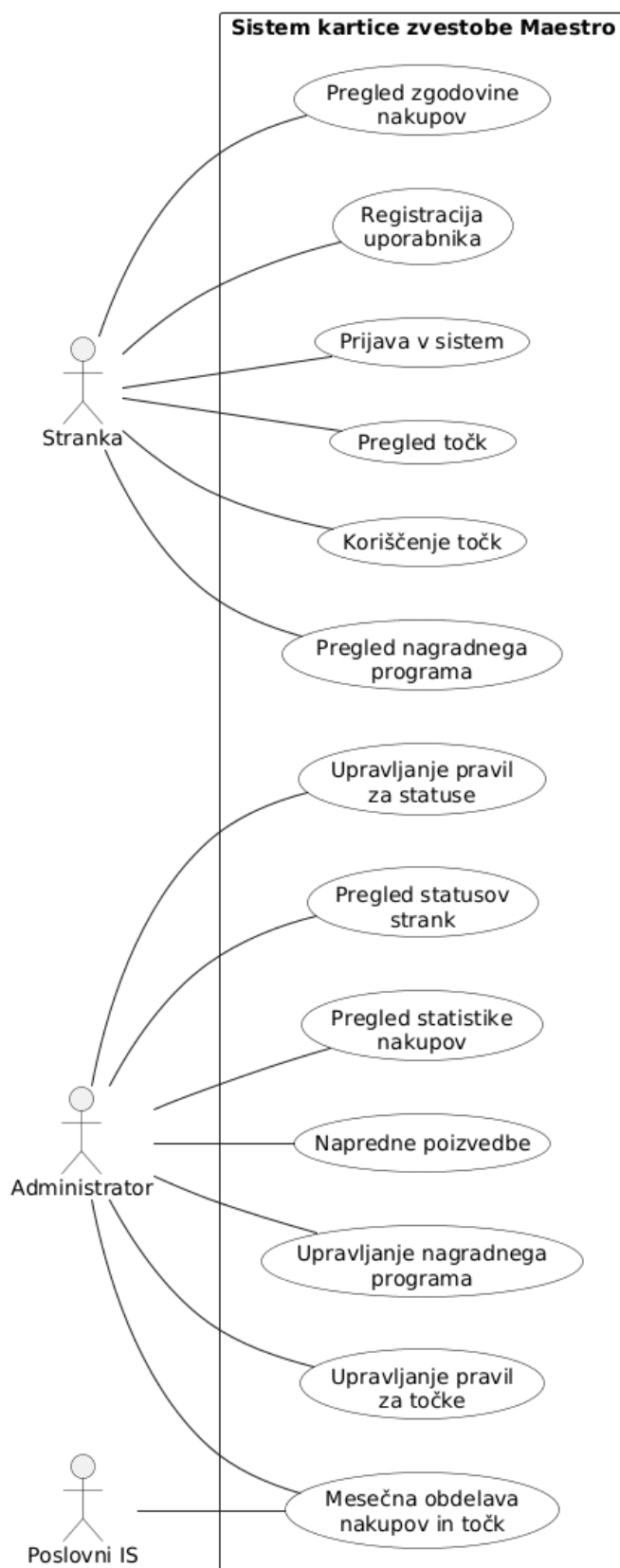
Diagram primerov uporabe
