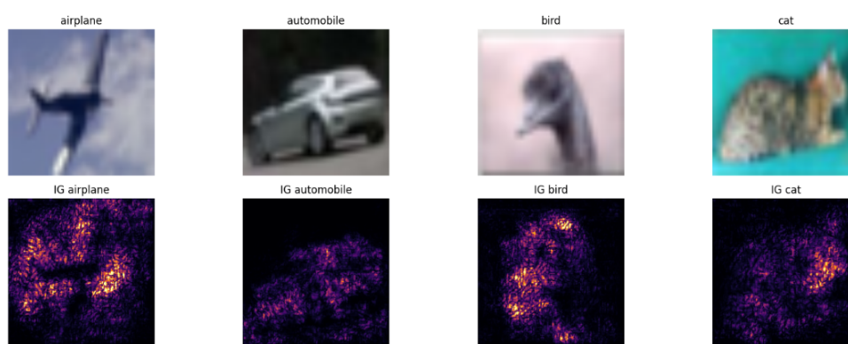
Rysunek 5.1. Mapy atrybucji Integrated Gradients dla obrazów niezaburzonych
