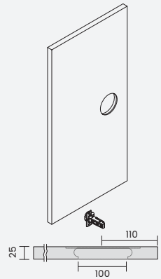
MLS.YX.0.07 圆月拉手 MLS.YX.0.07 Round Moon Handle
