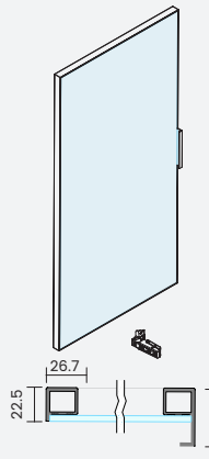
LB.SF.0.08 隐框玻璃门 ( 普通铰 ) LB.SF.0.08 Hidden Frame Glass Door (Ordinary Hinge)
