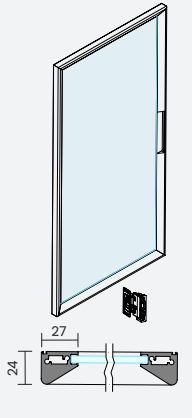
LB.SF.1.06 针式铰链玻璃门 LB.SF.1.06 Pin Hinged Glass Door
