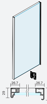
LB.SF.1.07 针式铰链玻璃门 LB.SF.1.07 Pin Hinged Glass Door
