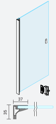
LB.SF.1.05 针式铰链玻璃门 LB.SF.1.05 Pin Hinged Glass Door
