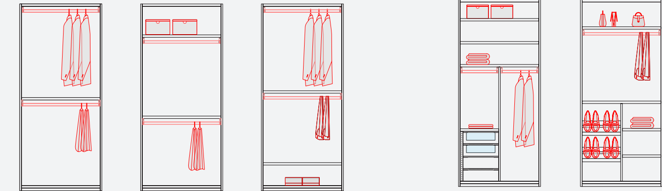
组合 1 Combination 1 组合 1.1 Combination 1.1 组合 1.2 Combination 1.2 组合 2 Combination 2 组合 2.1 Combination 2.1
