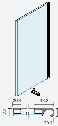
LB.DY.0.09 隐框 G 型拉手 ( 普通铰 ) LB.DY.0.09 Hidden Frame G-Shaped Handle(Ordinary Hinge)
