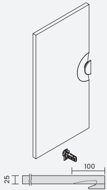
MLS.SX.0.08 扇形拉手 MLS.SX.0.08 Fan shaped handle
