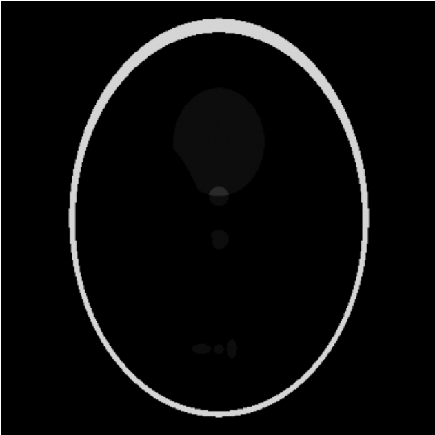
Bone Window C=400, W=1800
