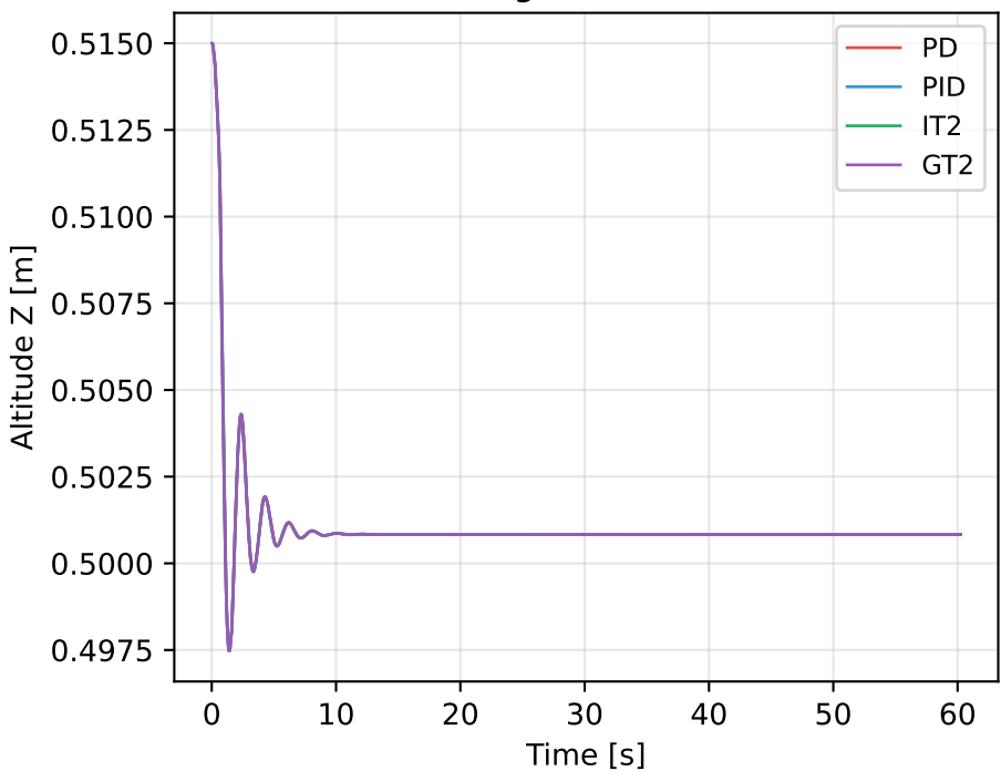
Altitude Holding (Z vs Time) - Phase 1
