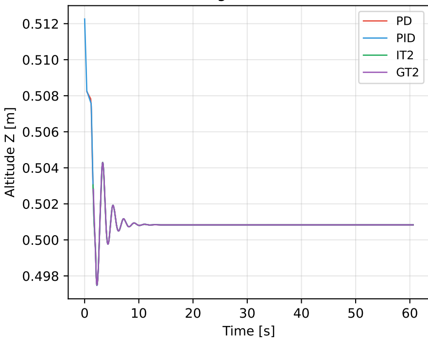
Altitude Holding (Z vs Time) - Phase 3
