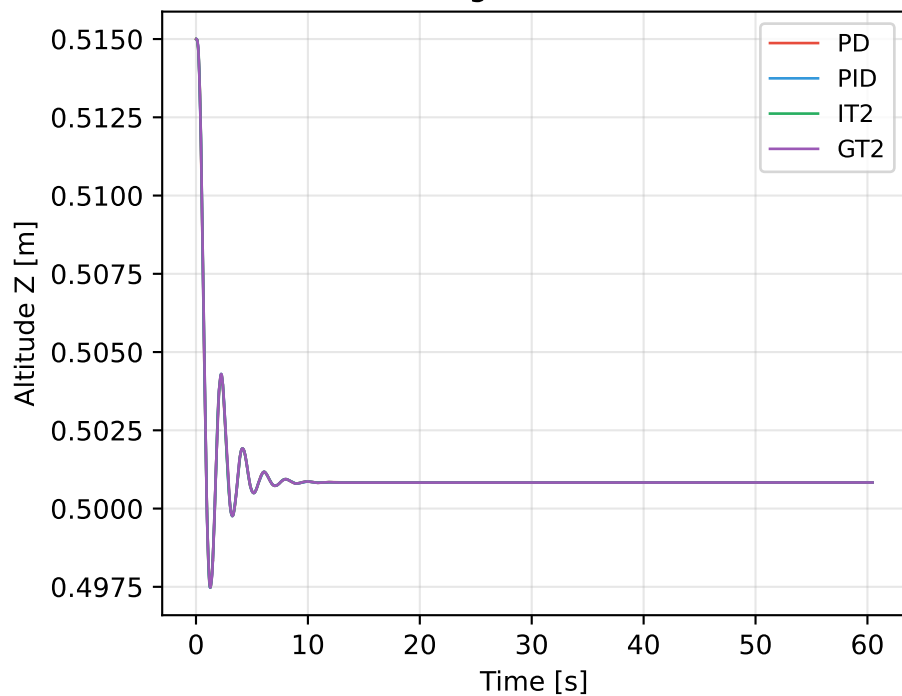
Altitude Holding (Z vs Time) - Phase 4
