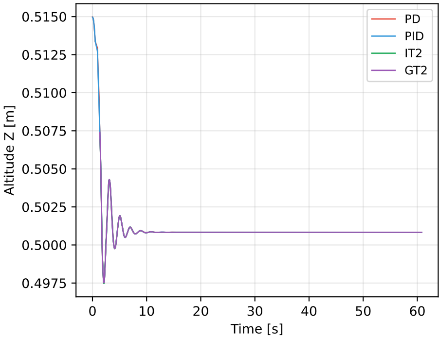
Altitude Holding (Z vs Time) - Phase 5
