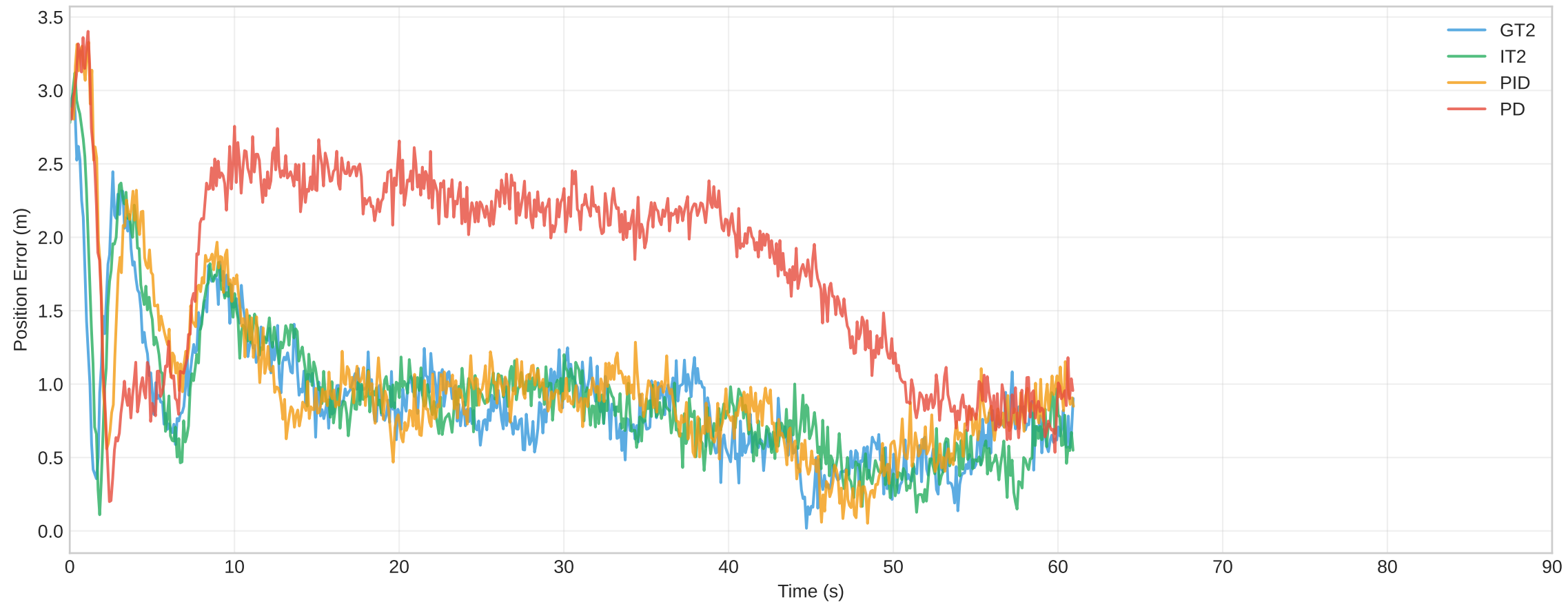
Phase 3: Turbulence (Von Karman) - Error Evolution
