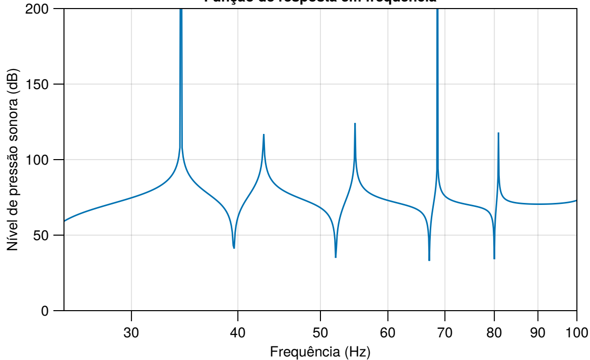
Função de resposta em frequência
