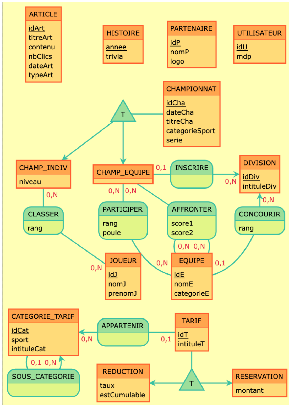
Figure 1 : Diagramme MCD de la base de données
