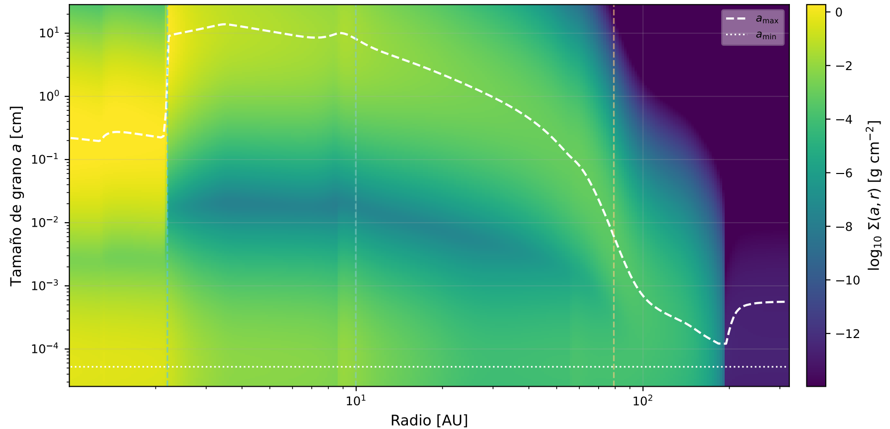
Distribución de tamaño de grano vs radio | t = 1.00\text{e}+05 yr
