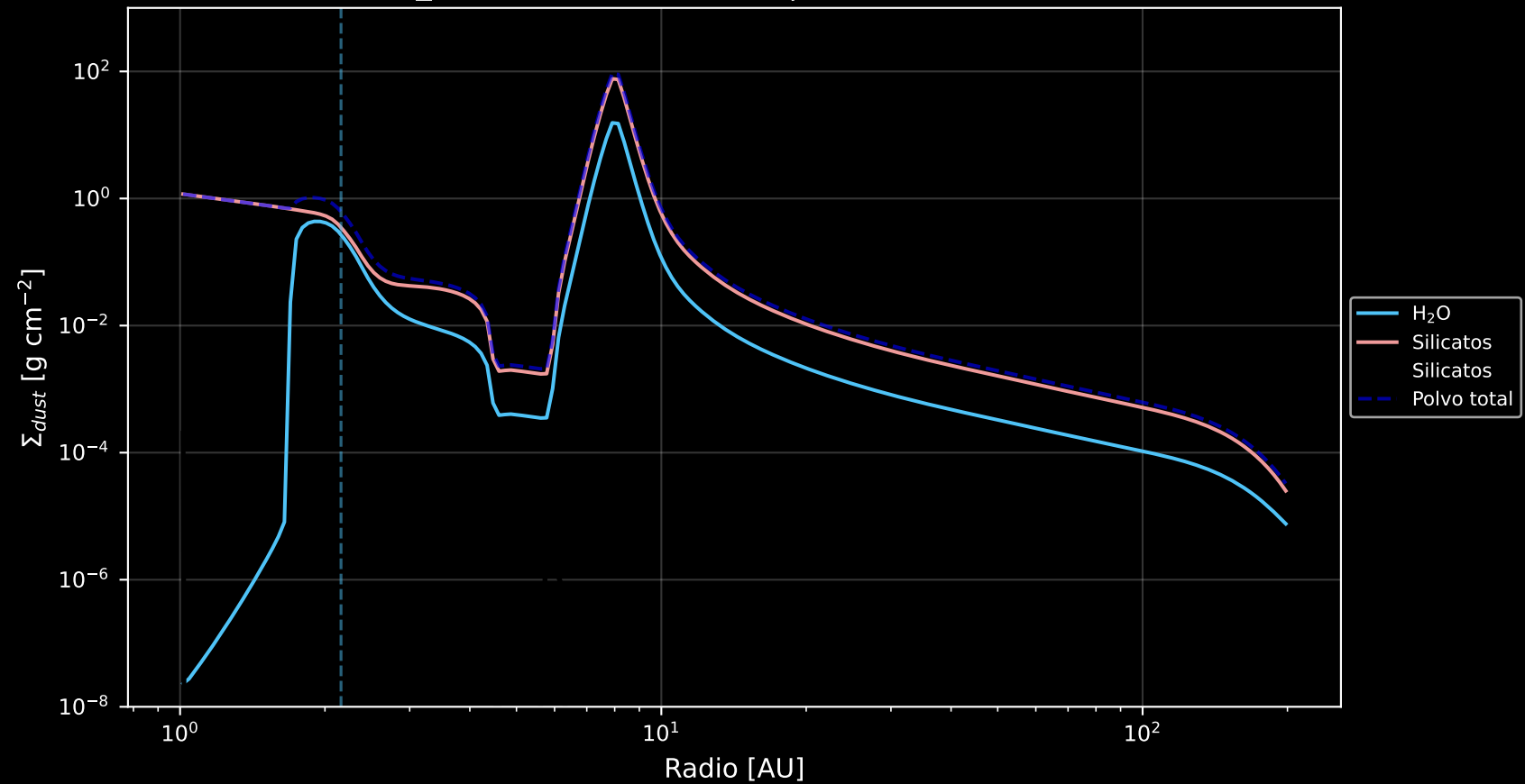
\Sigma_{dust} por componente | t = 1.00e+06 yr
