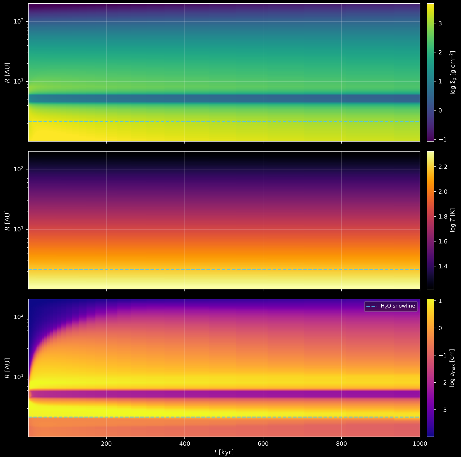
Diagrama Espacio-Tiempo R(t)
