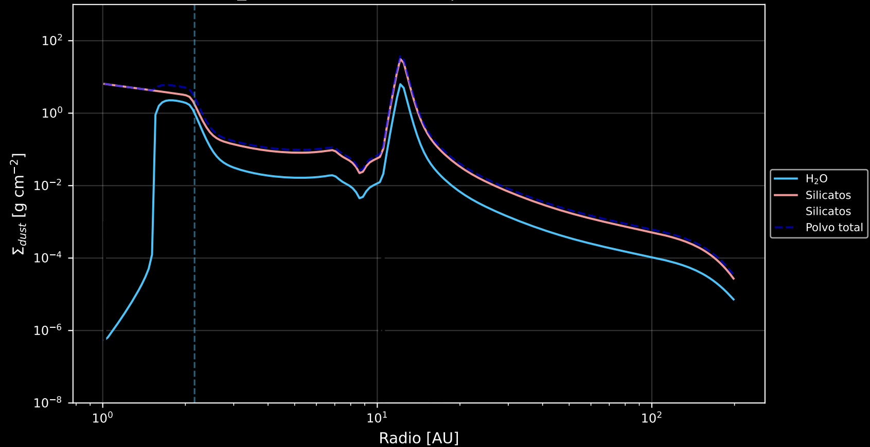
\Sigma_{\text{dust}} por componente | t = 1.00\text{e}+06 yr
