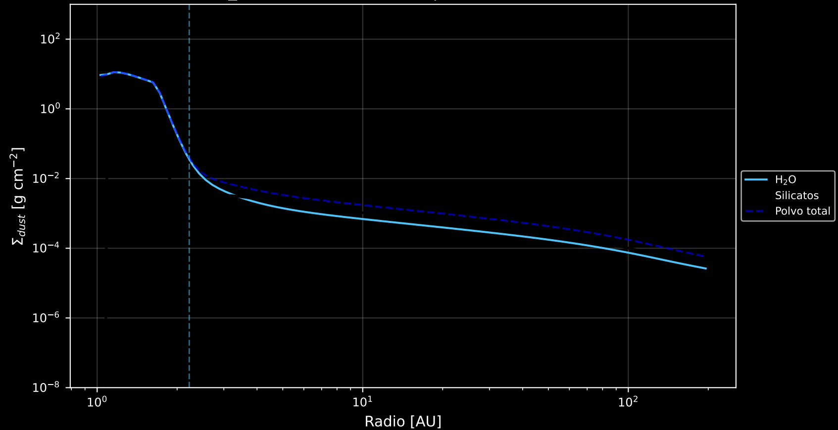
\Sigma_{\text{dust}} por componente | t = 1.00\text{e}+07 yr
