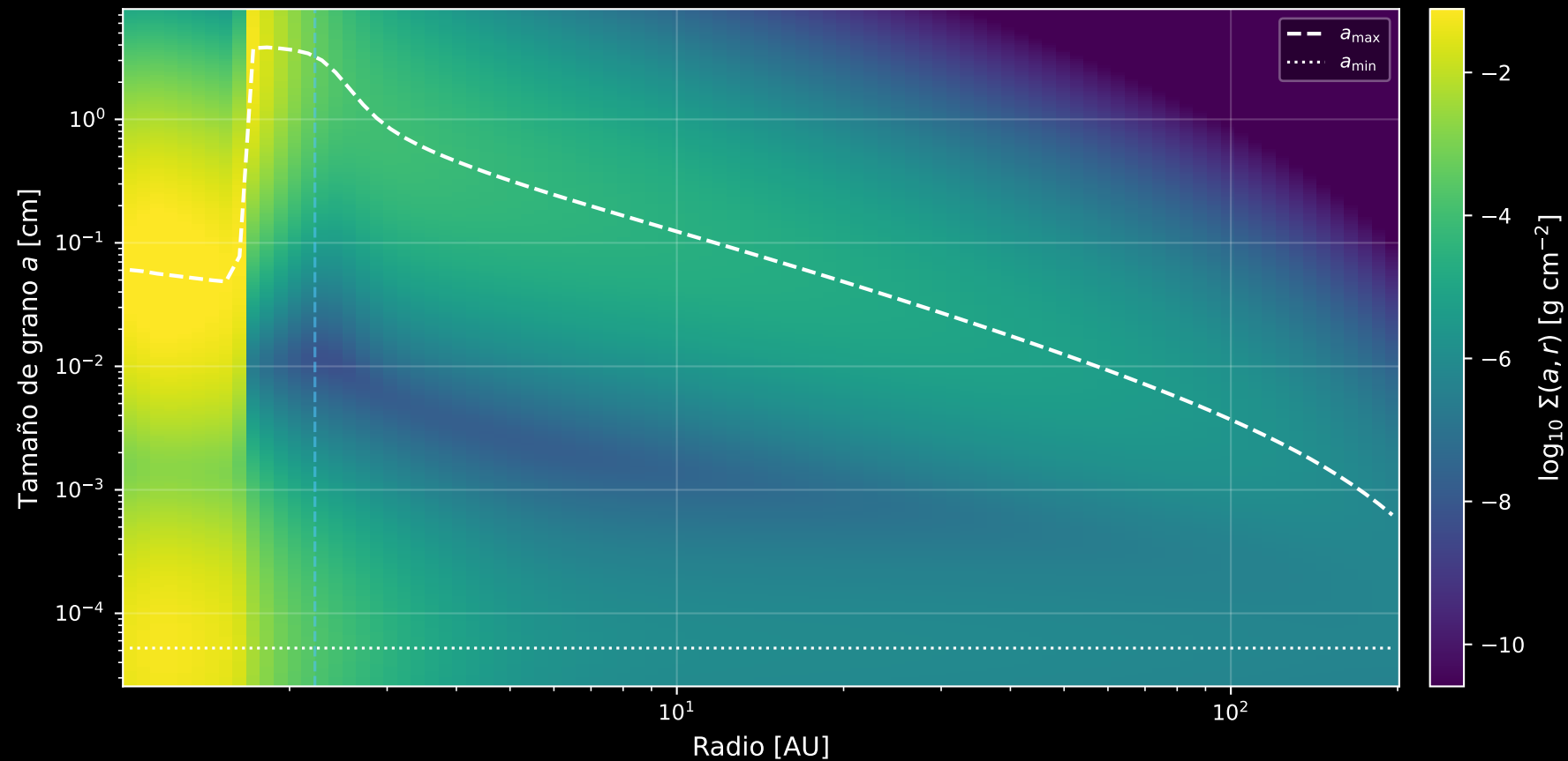
Distribución de tamaño de grano vs radio | t = 1.00\text{e}+07 yr
