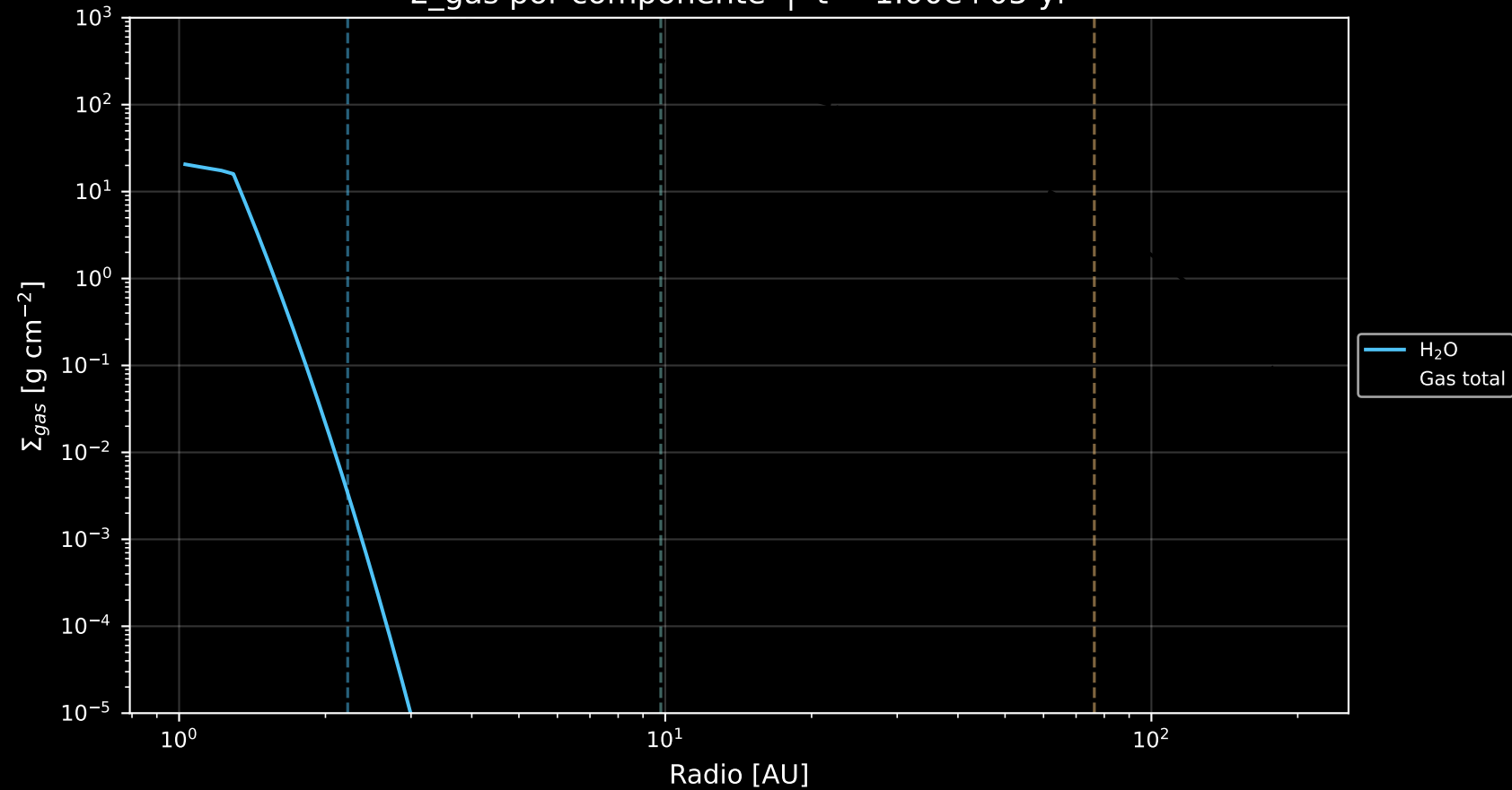
\Sigma_{\text{gas}} por componente | t = 1.00\text{e}+05 yr
