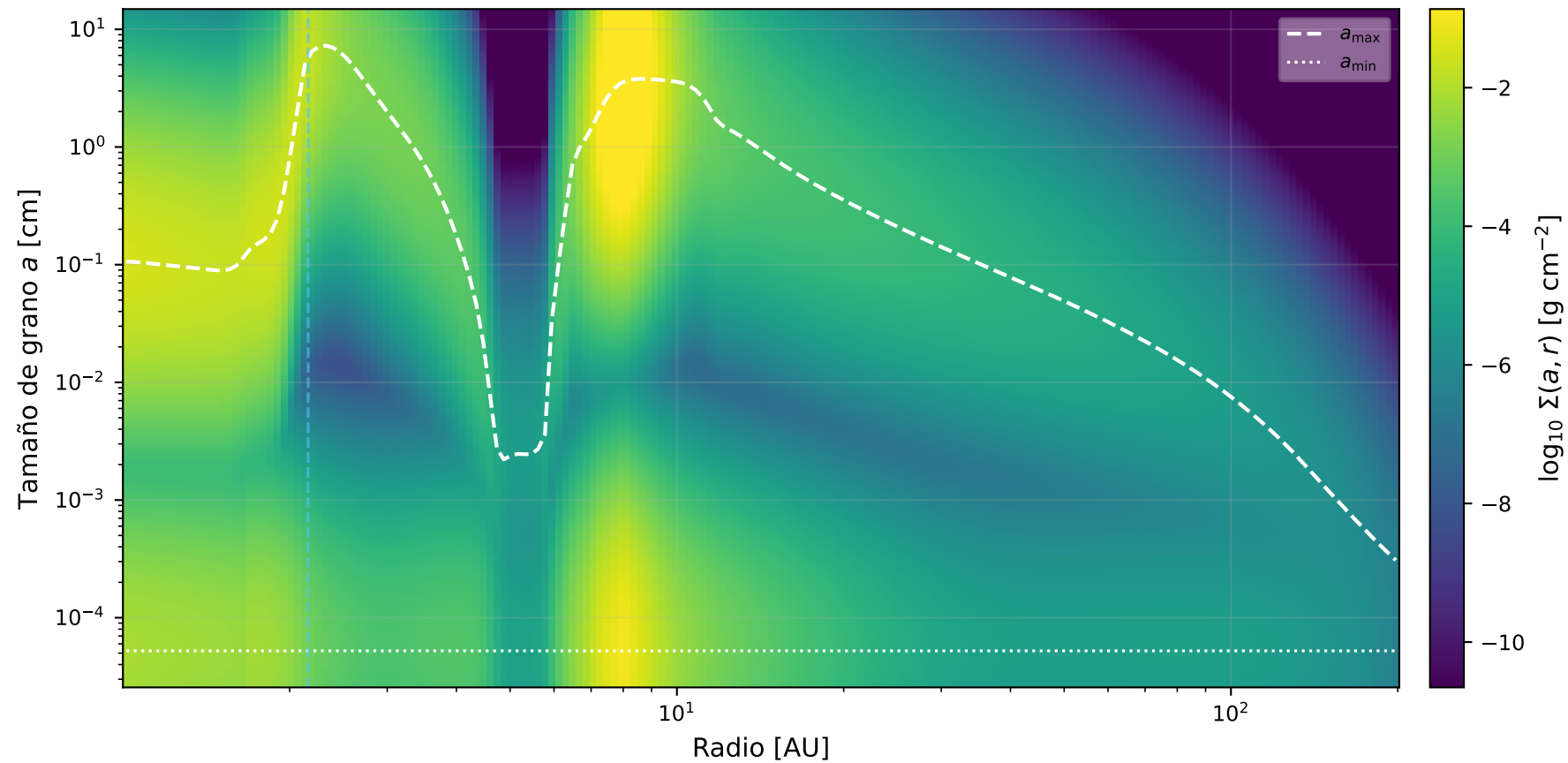
Distribución de tamaño de grano vs radio | t = 1.00\text{e}+06 yr
