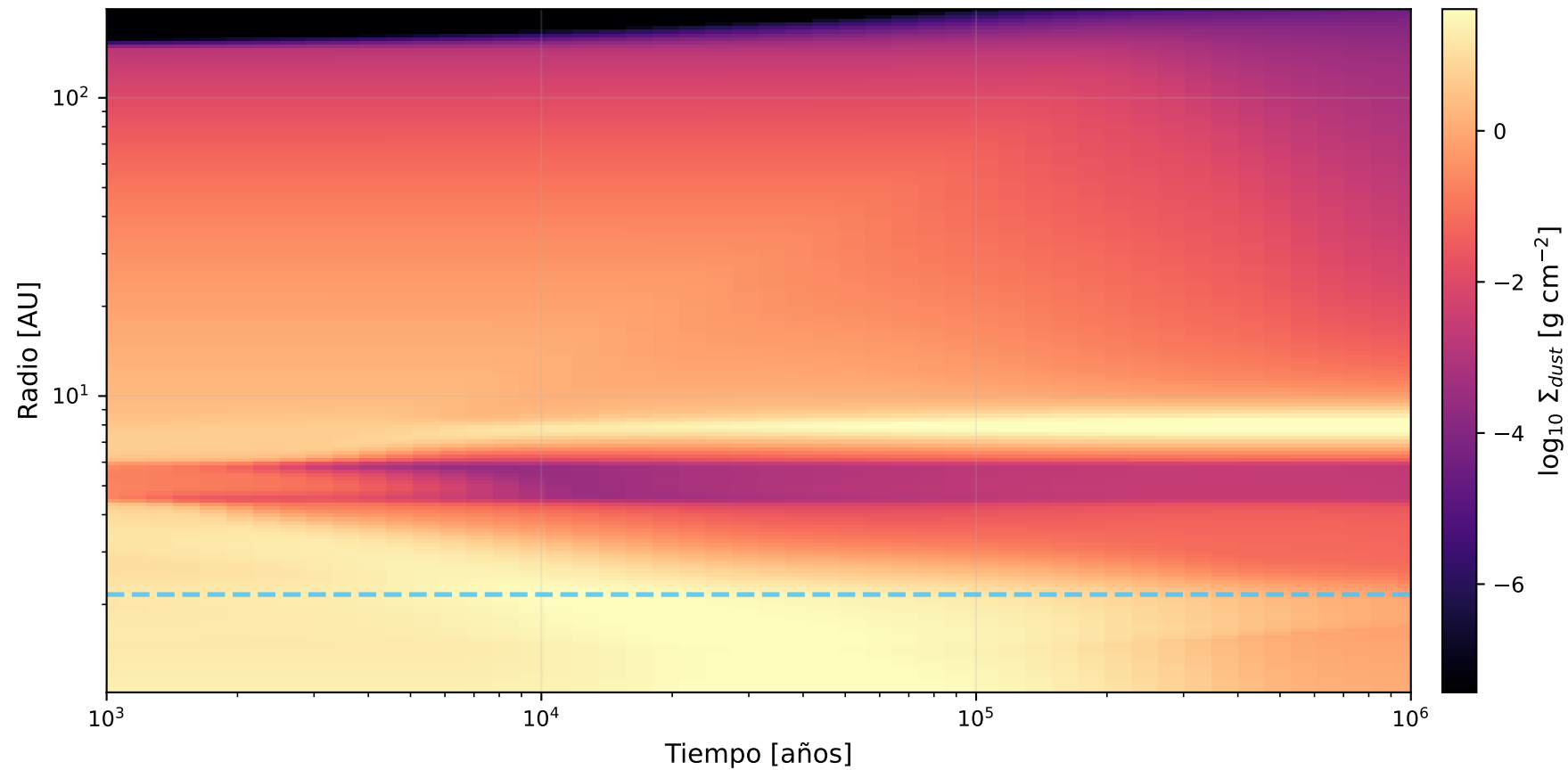
Diagrama Espacio-Tiempo: \Sigma_{dust}
