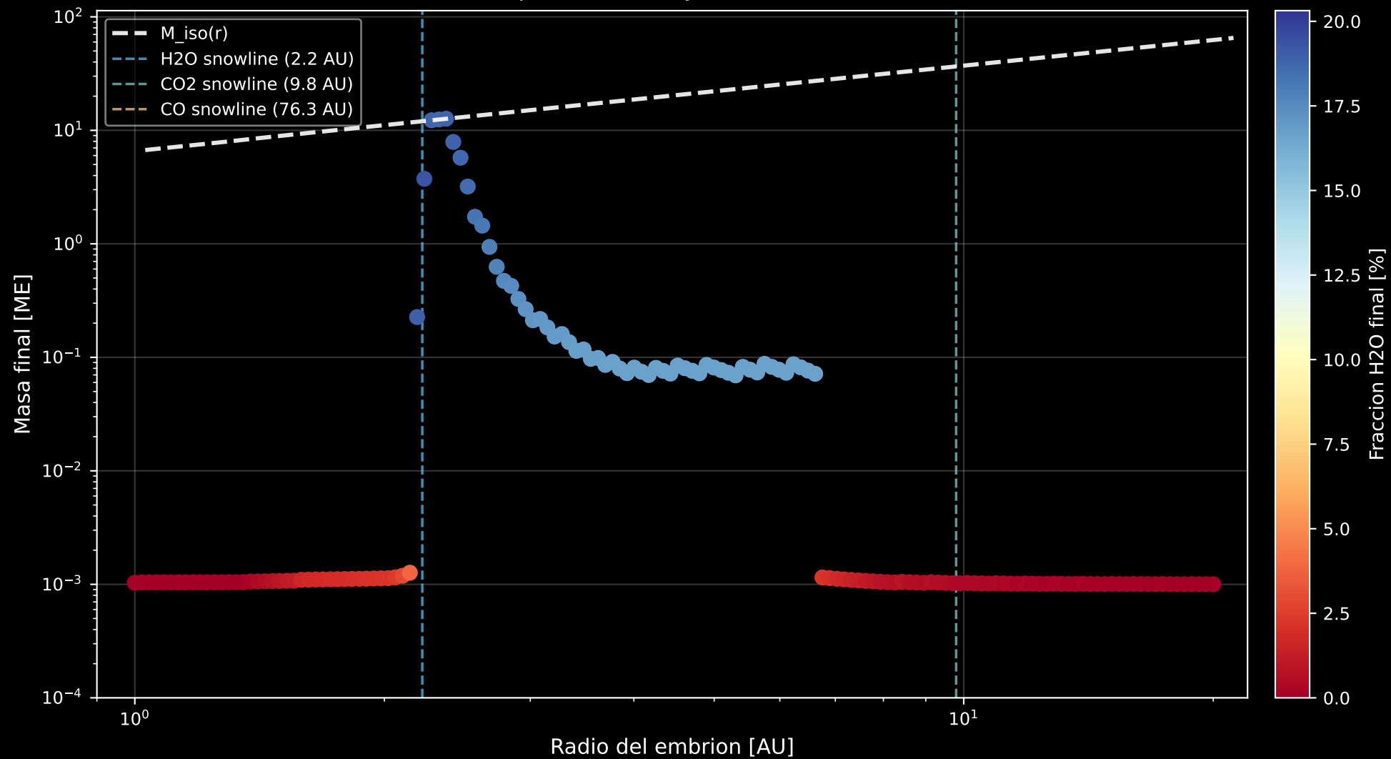
Waterworld Map: Masa final y fraccion de H2O vs radio
