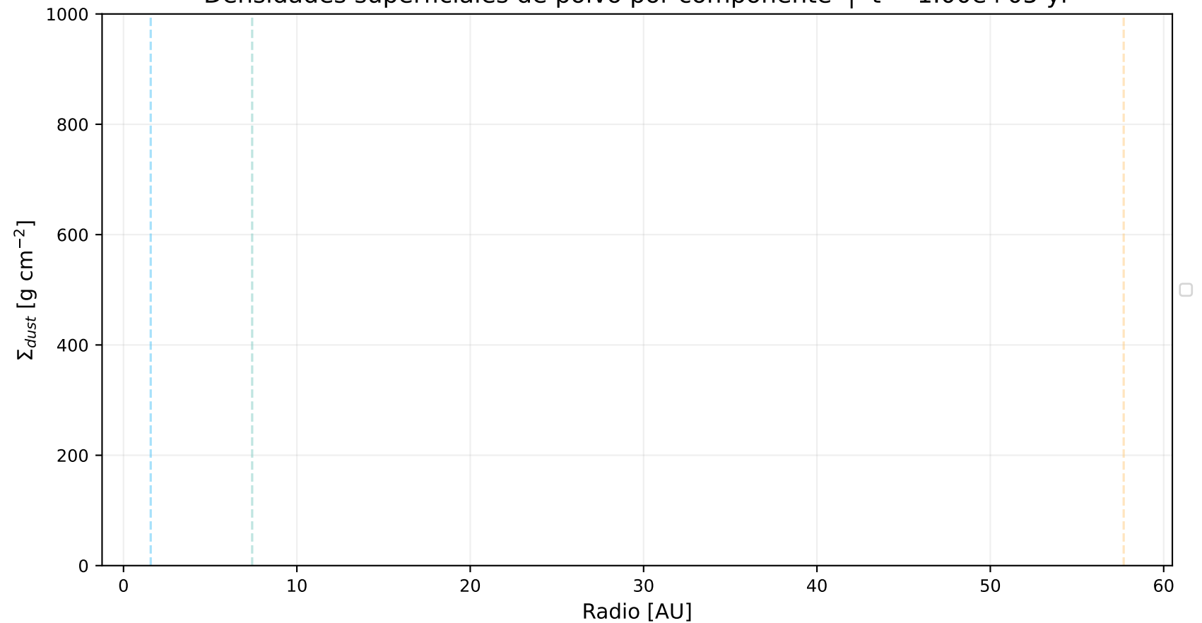
Densidades superficiales de polvo por componente | t = 1.00\text{e}+05 yr
