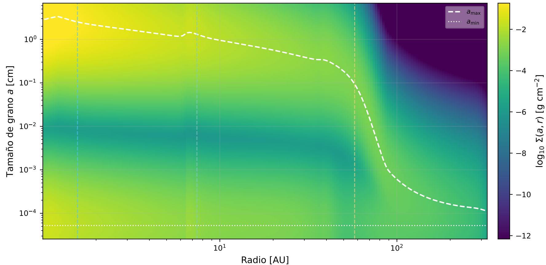
Distribución de tamaño de grano vs radio | t = 1.00\text{e}+05 yr
