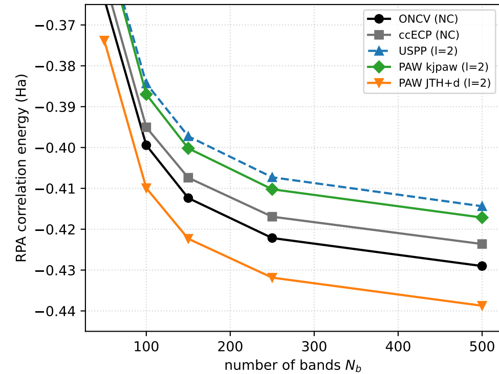
Si, 2×2×2 k-grid
