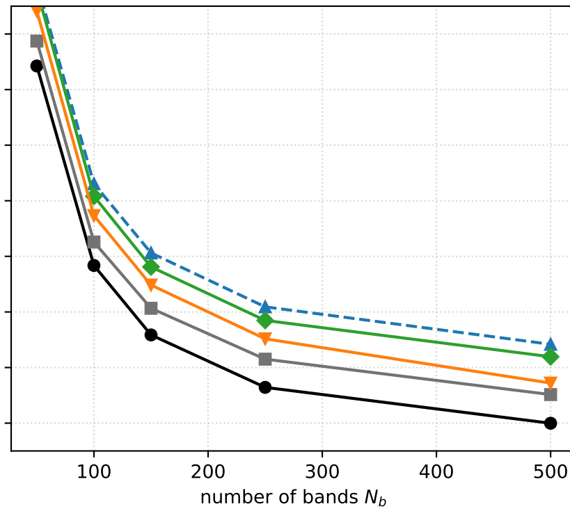
Si, 3×3×3 k-grid
