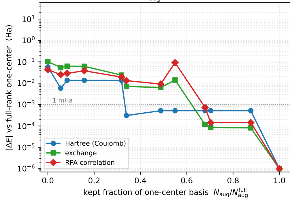
Si (kjpaw, no semicore)
