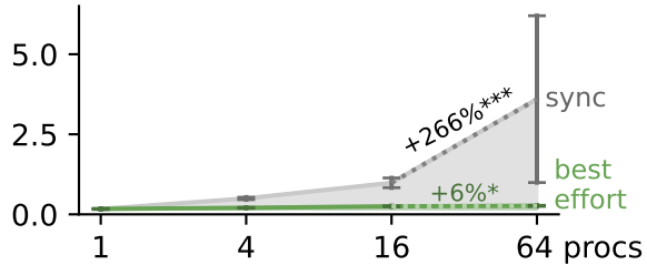
Graph Color (ms per update)
