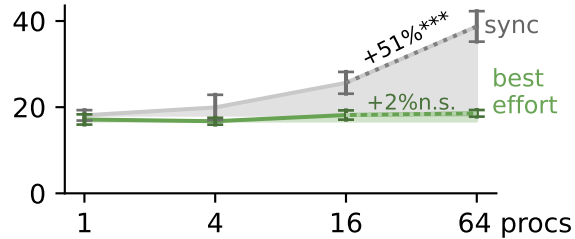
Digital Evo (ms per update)
