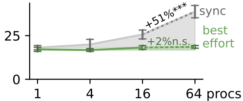
Digital Evo (ms per update)
