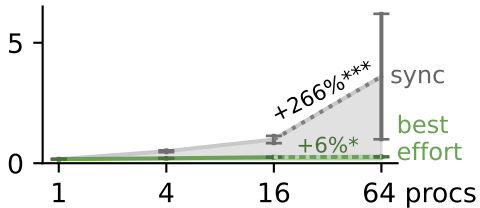
Graph Color (ms per update)
