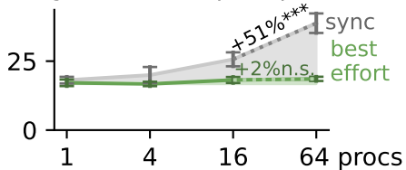
Digital Evo (ms per update)
