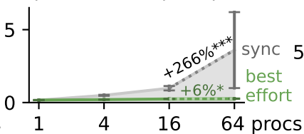
Graph Color (ms per update)
